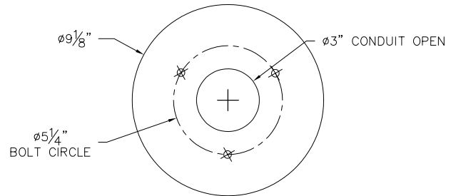
79 818 ANCHOR TEMPLATE
